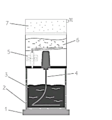
Рисунок 1 – Биореактор.
